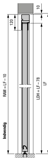
Separat dør med aluminium-standardkarm profiltype 2 Montering i åbningen
