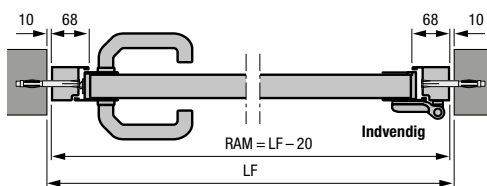
Separat dør med aluminium-standardkarm profiltype 2 Montering i åbningen
