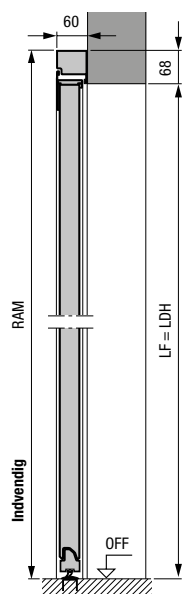
Separat dør med aluminium-standardkarm profiltype 2 Montering bag åbningen
