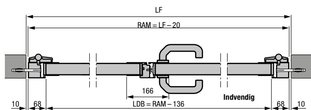
2-fløjet separat dør med aluminium-standardkarm profiltype 2 Montering i åbningen
