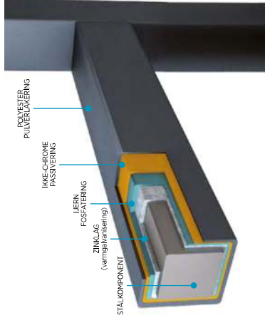
Tværsnit af et element sikret med DUPLEX systemet.
